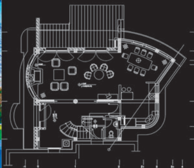
ПРИЗЕМЈЕ
