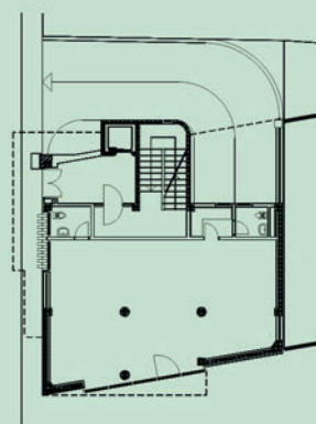
основа на приземје
