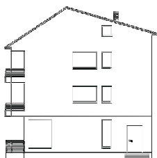
Фасади - постојечка состојба
