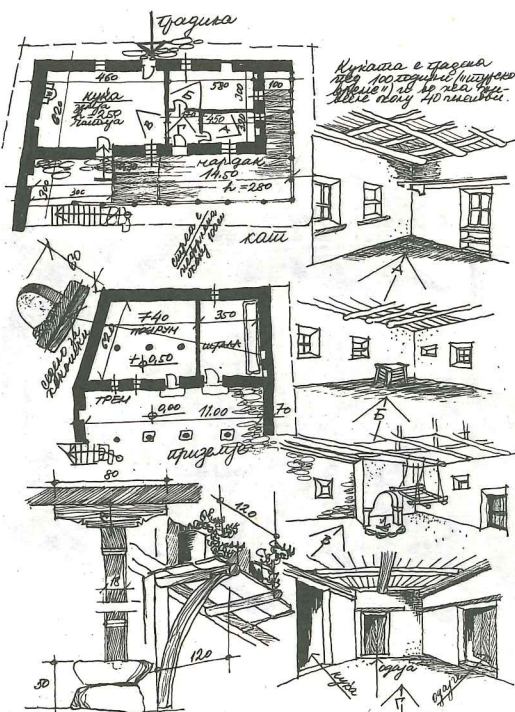
Куката на Цветко Кекенков со карактеристичен чардак во форма на буквата "Г"
