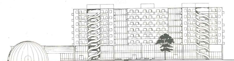
ЈУЖНА ФАСАДА M=1:200
